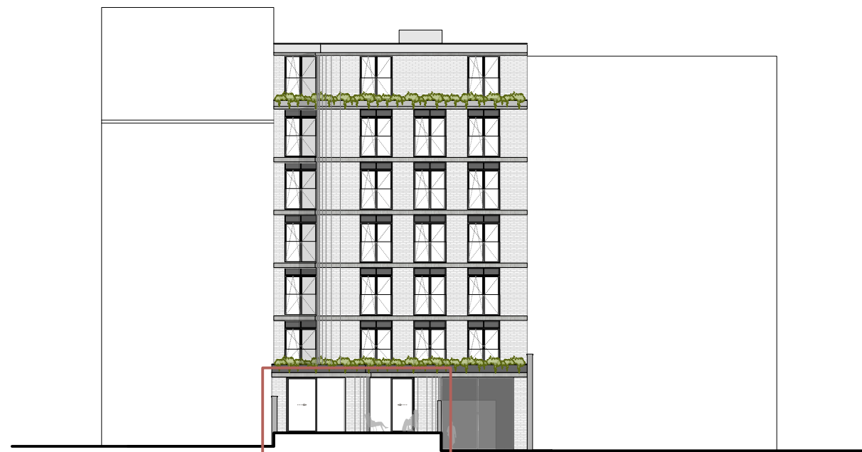
Achtergevel
